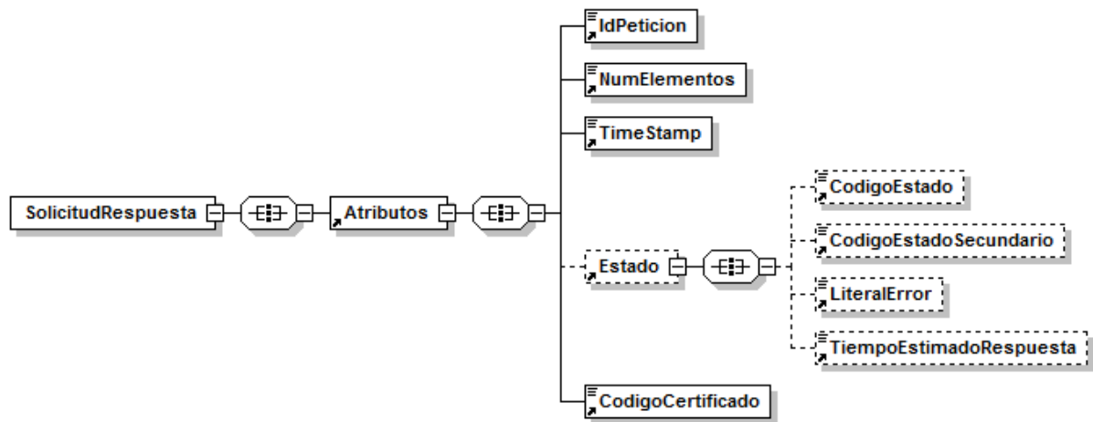
Figura 11. Diagrama del mensaje SolicitudRespuesta del Servicio
