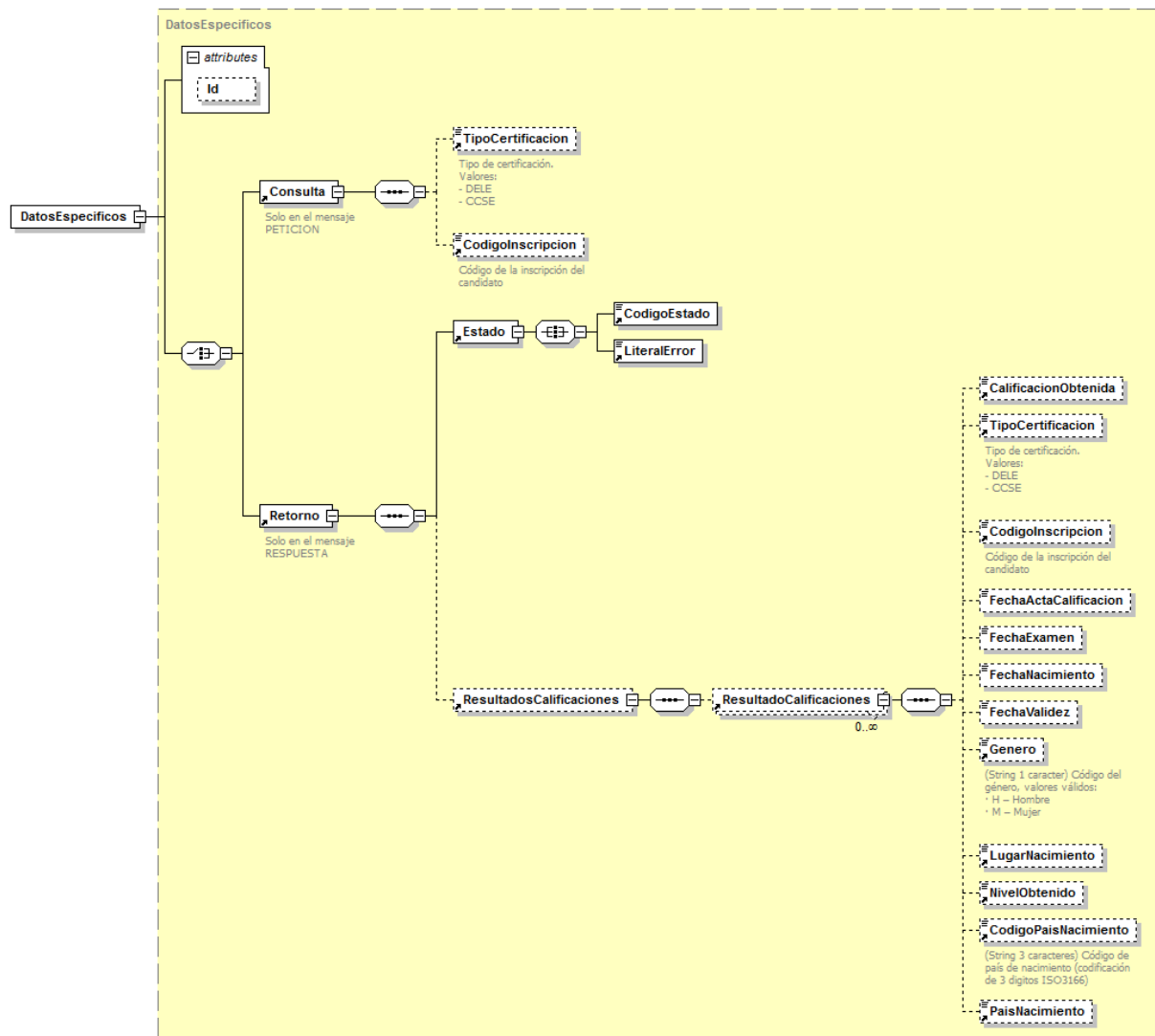
Figura 9. Diagrama de Datos Especificos de Respuesta del Servicio
