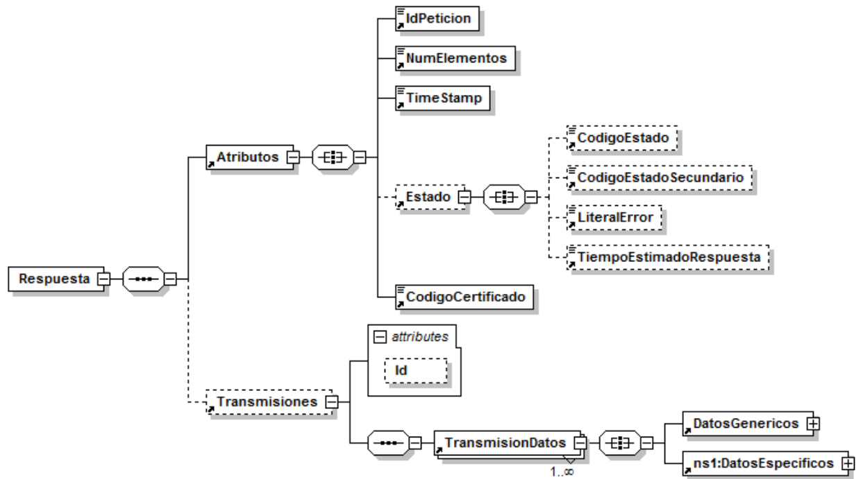
Figura 5 Mensaje de Respuesta al servicio de Consulta de subsistencia de poderes notariales
