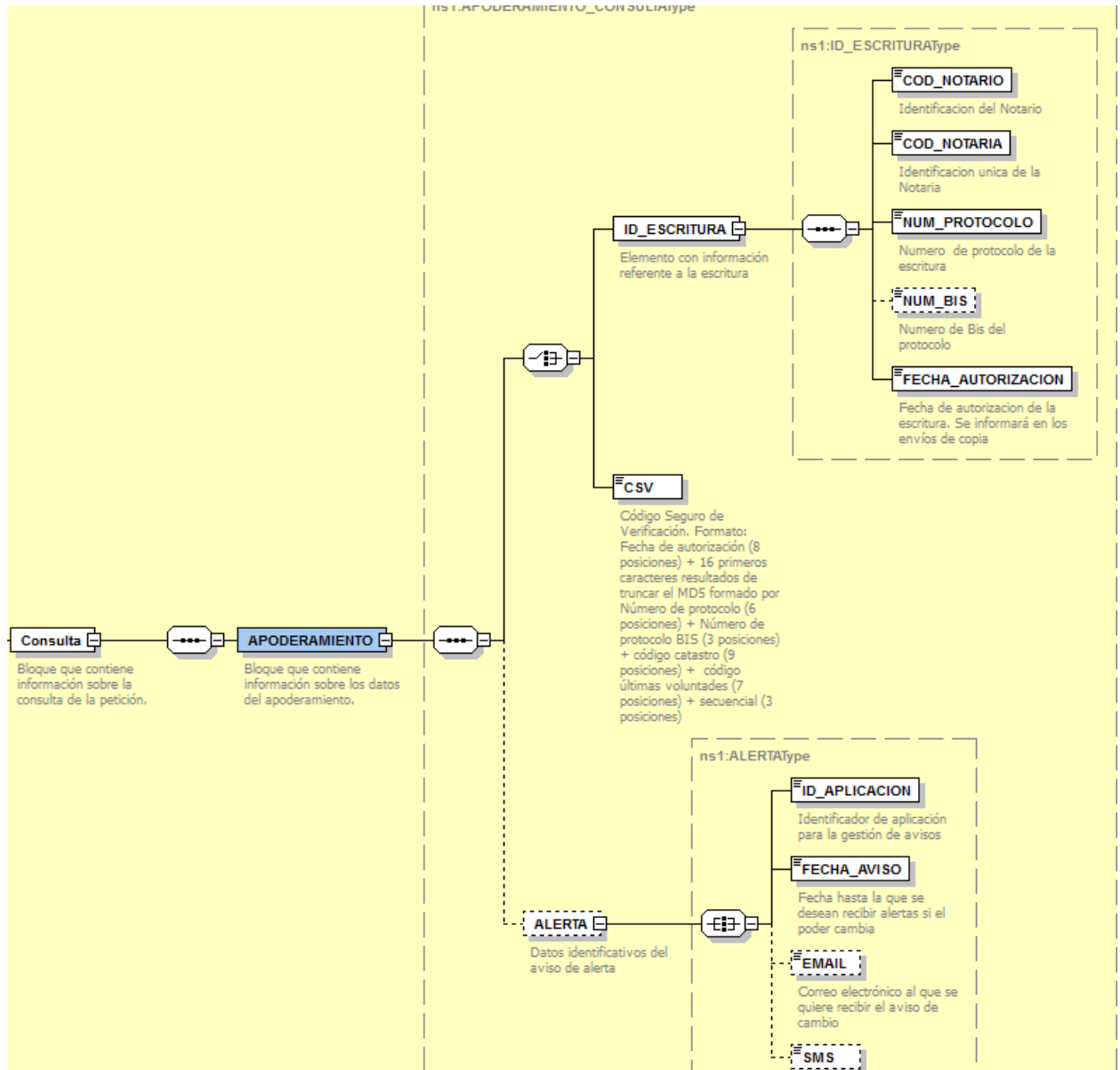
Figura 8 Datos Específicos para la Petici3n del Servicio de Consulta de Subsistencia – Elemento APODERAMIENTO
