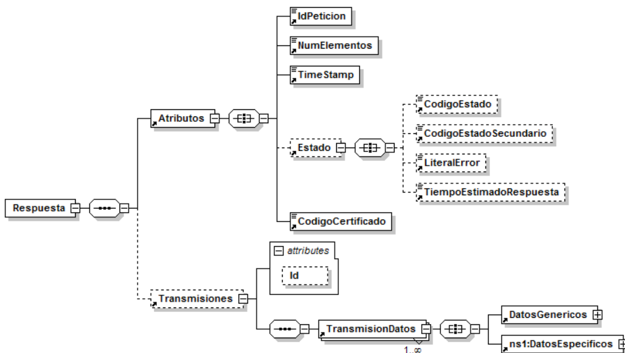
Figura 5 Mensaje de Respuesta al servicio de Consulta de Copia Simple
