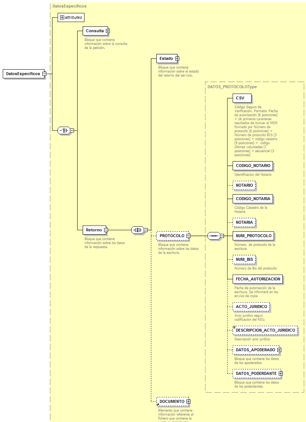
Figura 9 Datos específicos correspondiente a la respuesta del Servicio de Consulta de Copia Simple - Elemento PROCOLO
