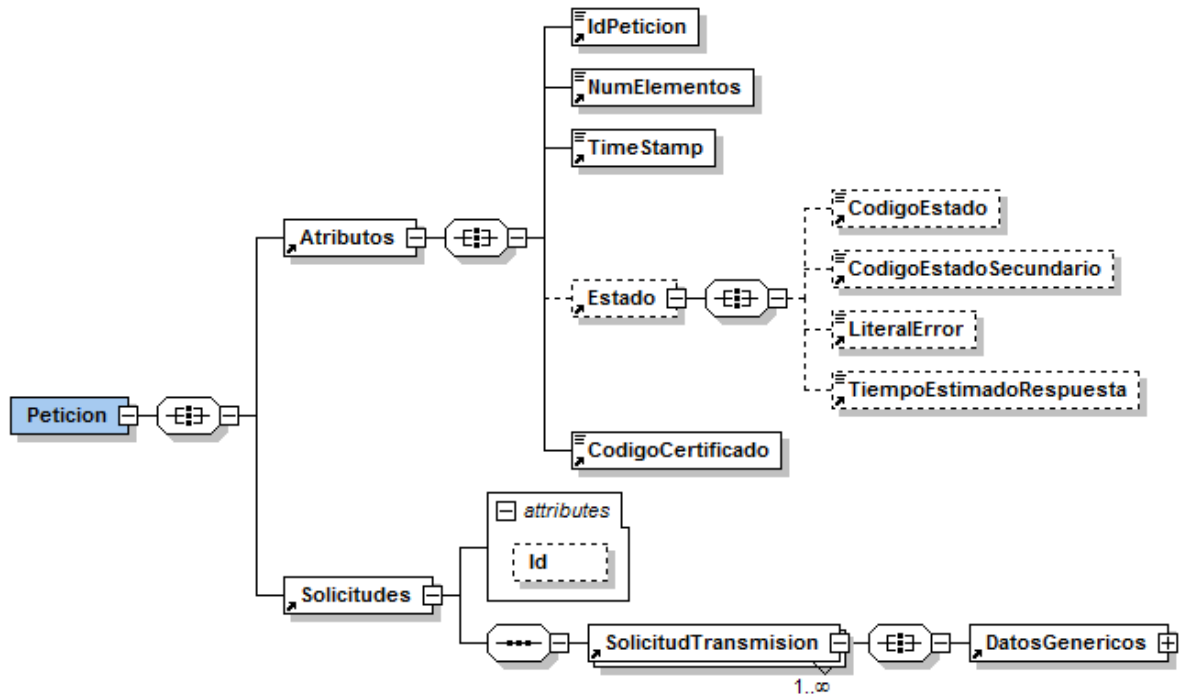
Figura 5.- Mensaje de petición al Servicio de Consulta de Nacimiento
