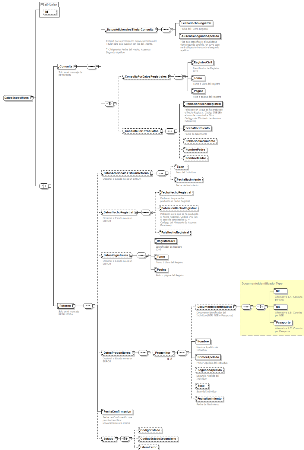
Figura 9.- Datos Especificos del Servicio de Consulta de Nacimiento
