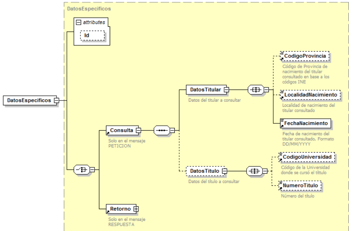
Figura 7.- Diagrama de Datos Específicos de Consulta del Servicio
