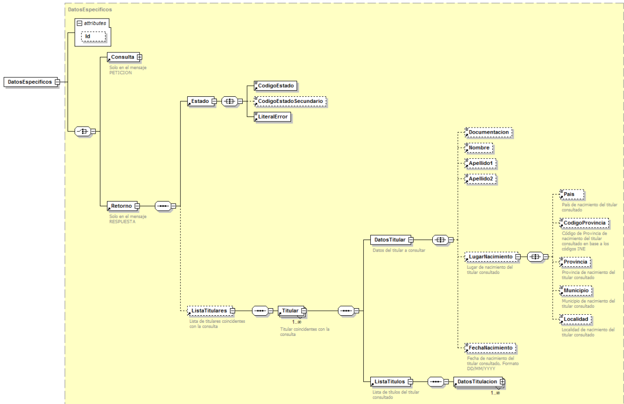
Figura 8.- Diagrama de Datos Específicos de Respuesta del servicio
