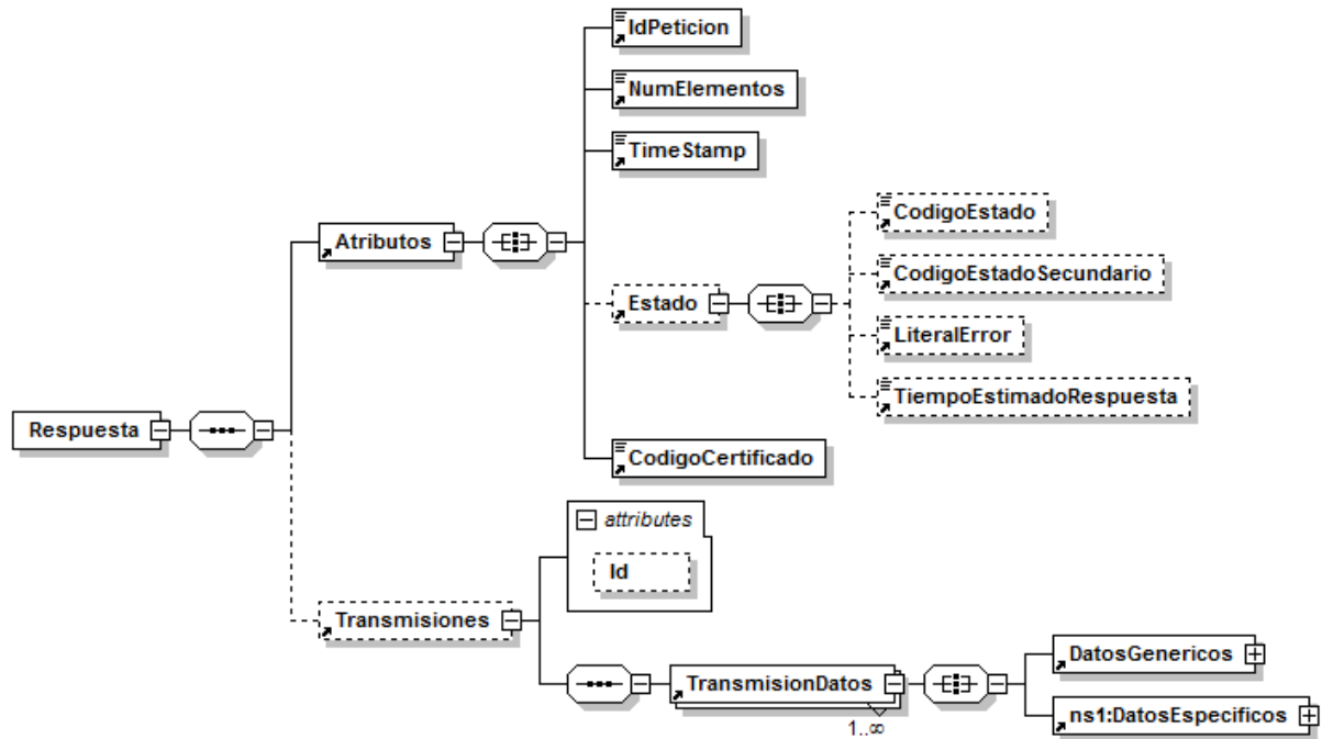
Figura 4. Diagrama de la rama DatosGenericos del mensaje de respuesta del Servicio
