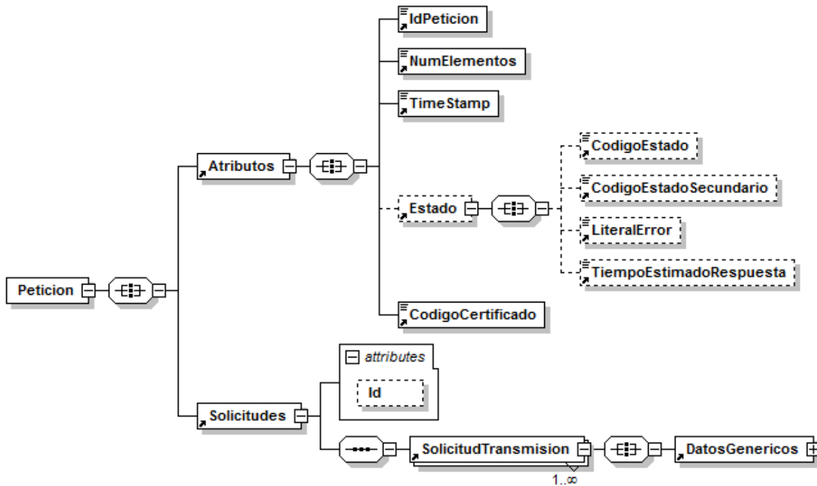
Figura 2. Diagrama del mensaje de petición del servicio
